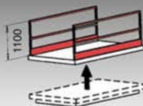
Schutzgeländer
