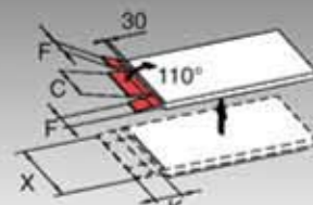
Überfahrblech
